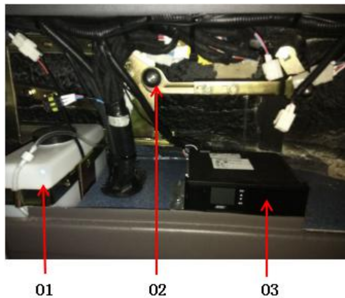
图 4.2.1 驾驶平台下舱
