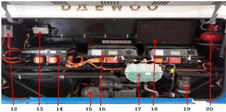
图 3.2.1 左后侧电器元件舱
