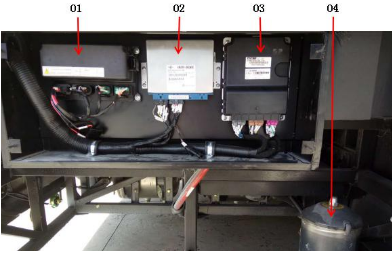
图 3.3.1 驾驶平台下舱
