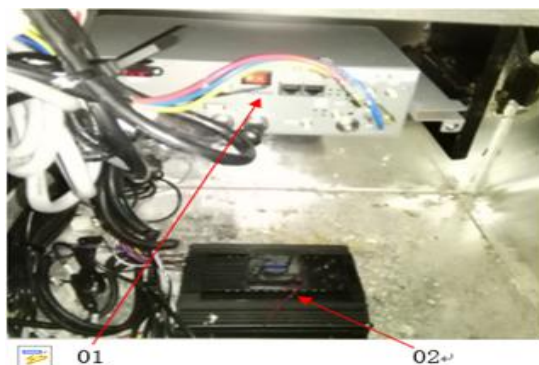
图 4.4.1 DVR 舱
