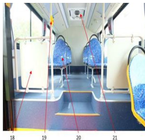
图 4.1.4 车内布局 4
