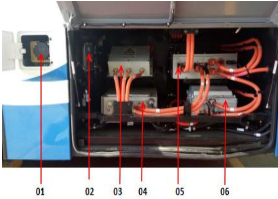
图 3.2.1 左后侧电器元件舱
