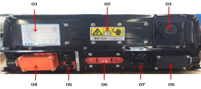
图 6.2.2.1 动力电池
