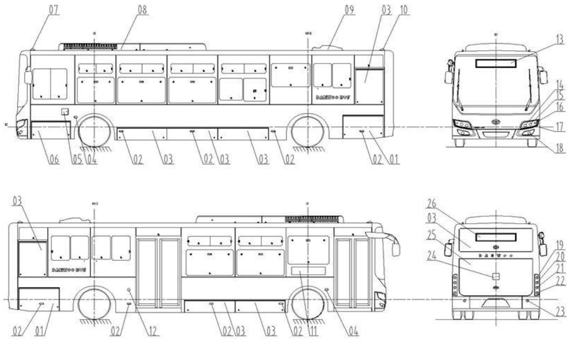
图 3.1.1 整车外观布局
