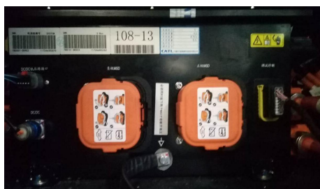
图 6.2.3.1 BMS 及维修开关位置
