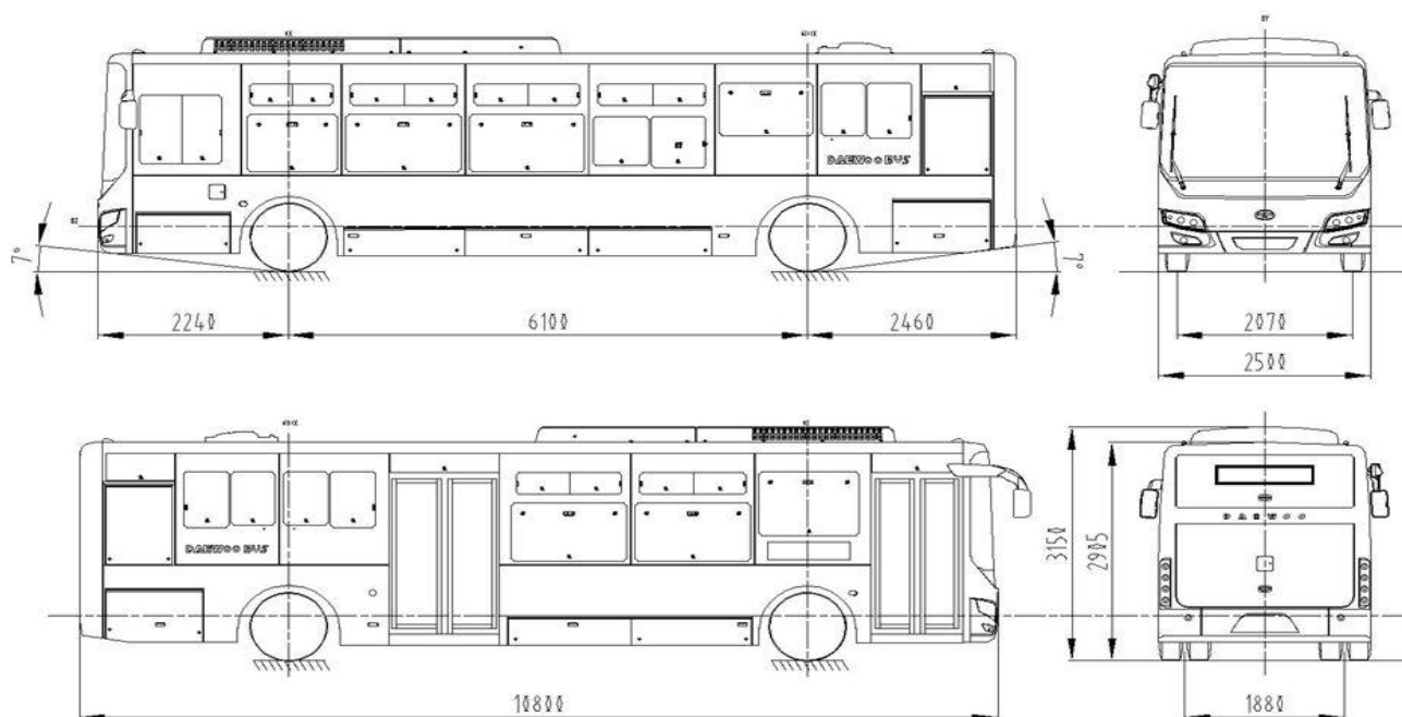
图 2.1.1 车辆外形尺寸
