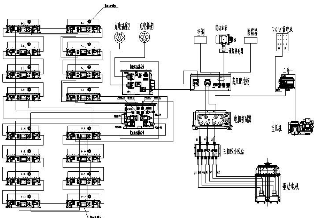
6.1.1 高压原理图
