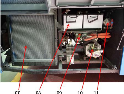
图 3.2.2 右后侧电器元件舱
