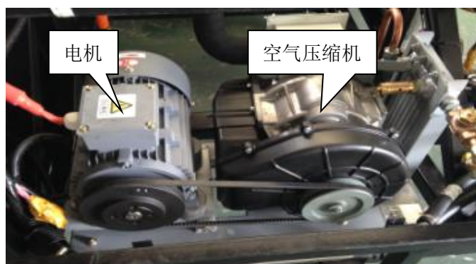
图 6.2.9.1 电动气泵
